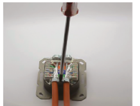
Schelle für Abschirmung festziehen Tighten screen clamp
